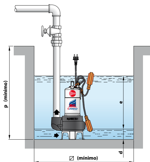
Instalación típica
