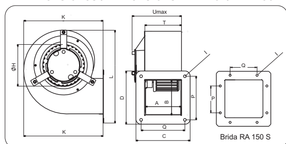
Dimensiones / Dimensions RH 200
