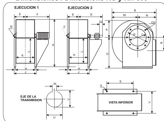
Dimensiones / Dimensions RG y RH 600
