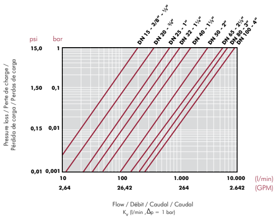
Pressure loss diagram Diagramme de perte de charge Diagrama de pérdidas de carga Diagrama das perdas de carga
