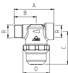
ATTACCO MF
