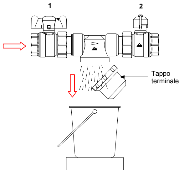
Fig. 1: Nell'immagine sopra riportata, si mostra come deve essere eseguita la manutenzione del filtro di linea per la pulizia / sostituzione della cartuccia filtrante.
