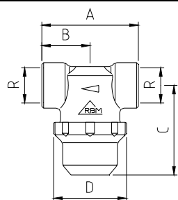
ATTACCO FF
