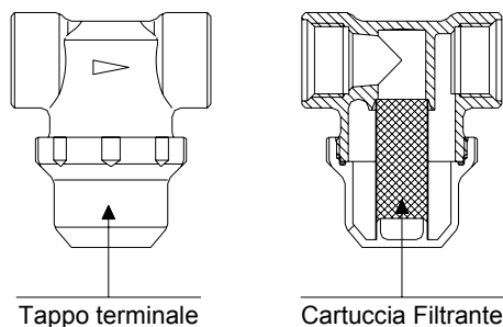
Fig. 2: Sotto viene riportato il filtro di linea con indicazione dei suoi componenti strutturali.
