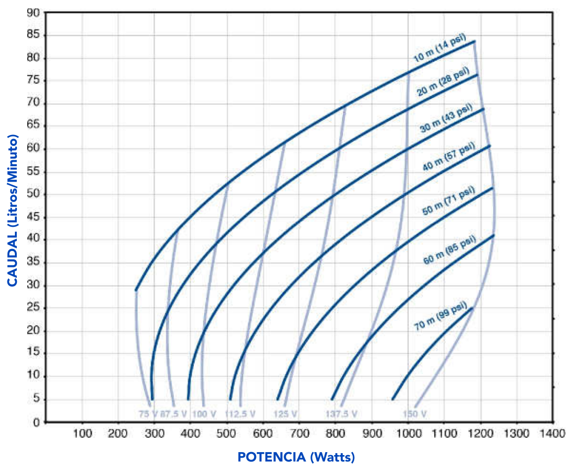
45 FDSP - 0.75 HP
