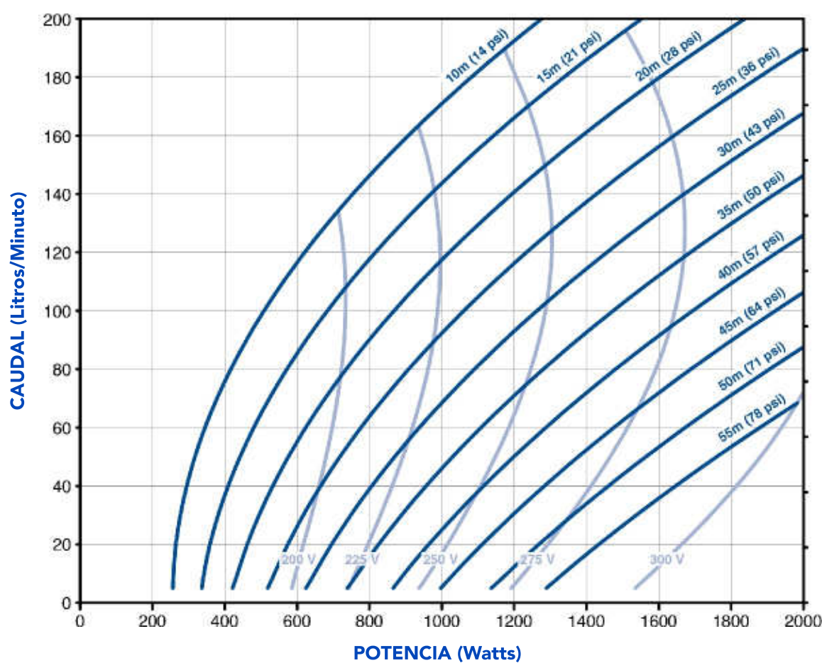
150 FDSP - 1.5 HP
