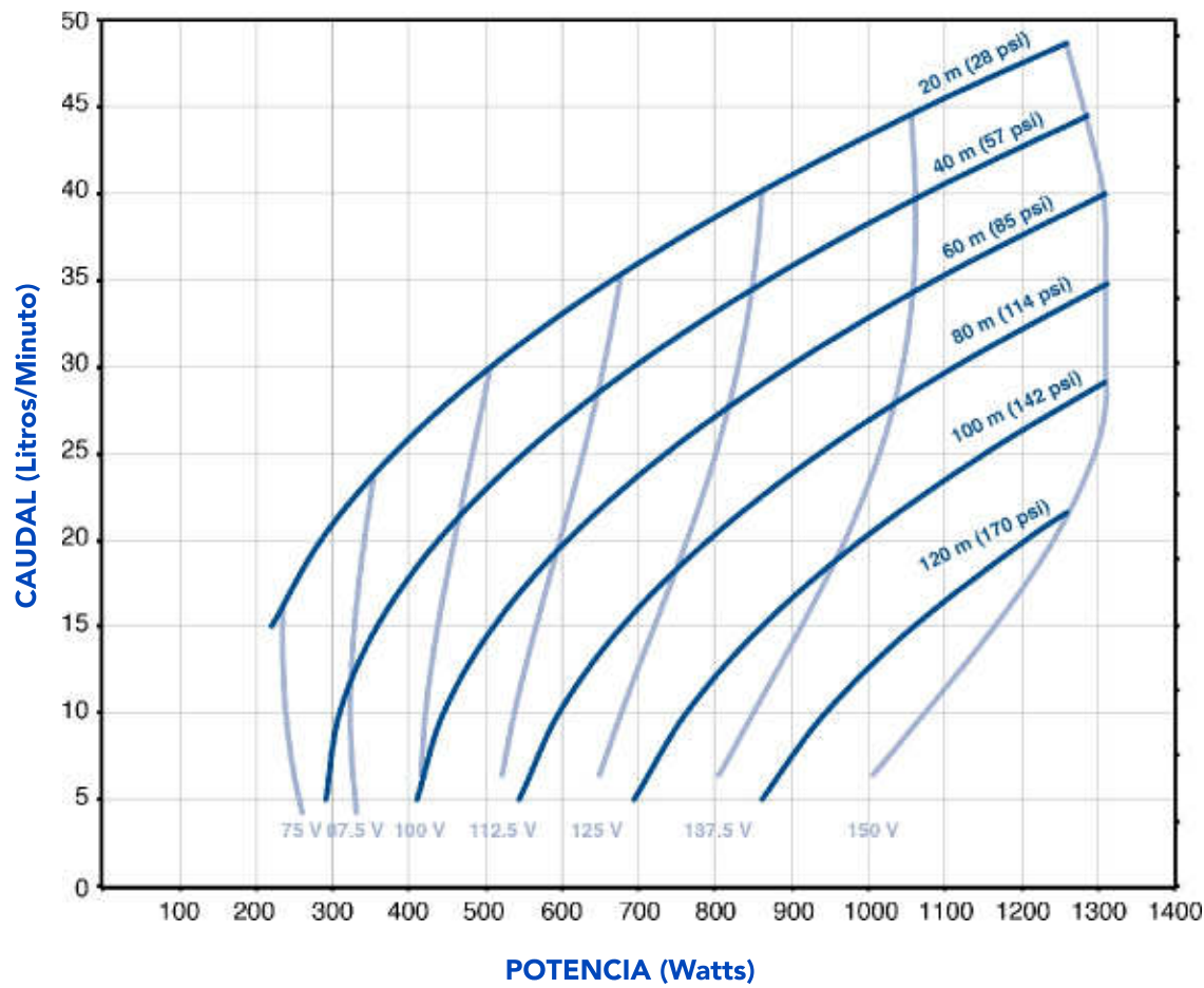
30 FDSP - 0.75 HP
