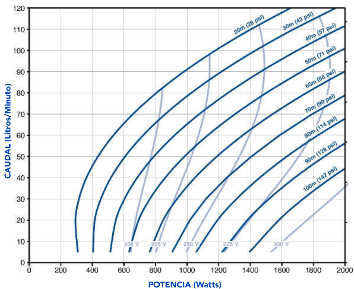
70 FDSP - 1.5 HP
