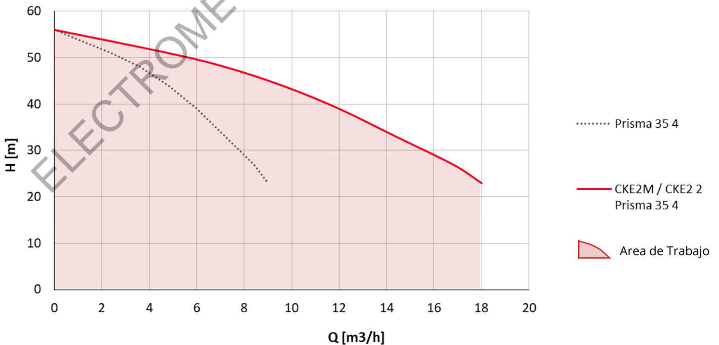
CKE 2M / CKE2 Prisma 35 4
